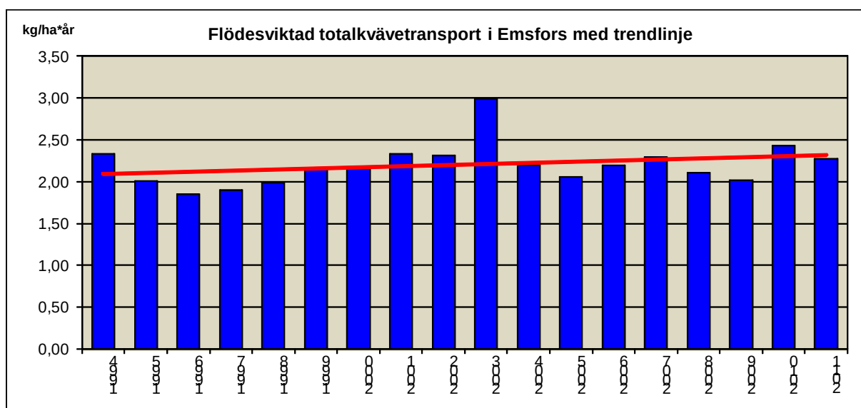
Figur 11. Årlig kvävetransport i Emsfors
