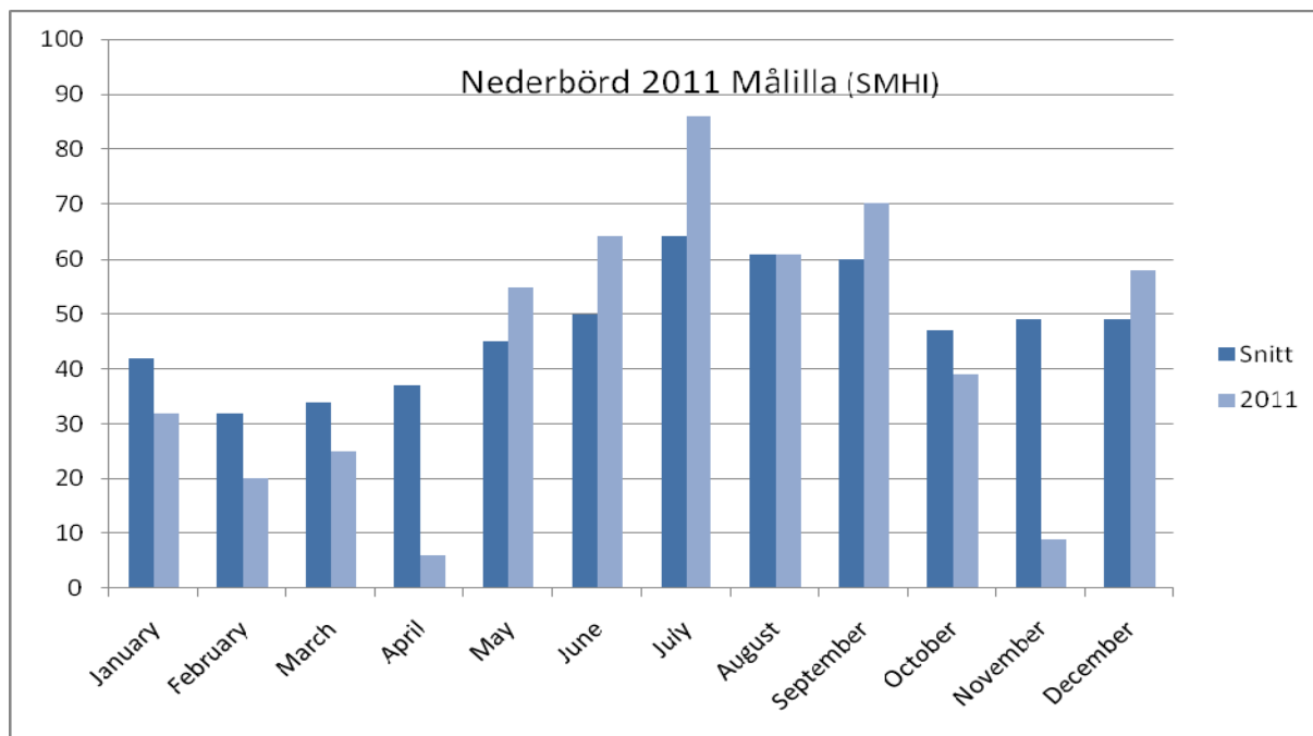
Figur 6. Nederbörd i Målilla 2011enligt SMHI. (Snitt 1961 – 1990)
