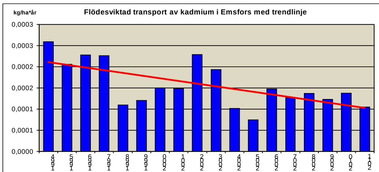
Figur 12. Flödesviktad transport av kadmium i Emsfors med trendlinje kg/ha och år
