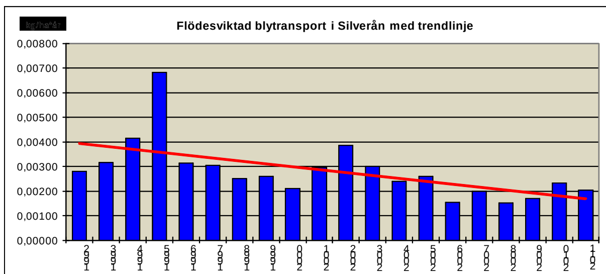
Figur 13. Flödesviktad transport av bly i Silverån nedströms Hulingen med trendlinje kg/ha och år
