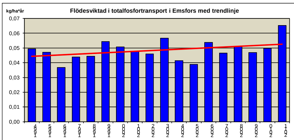
Figur 10. Årlig fosfortransport i Emsfors
