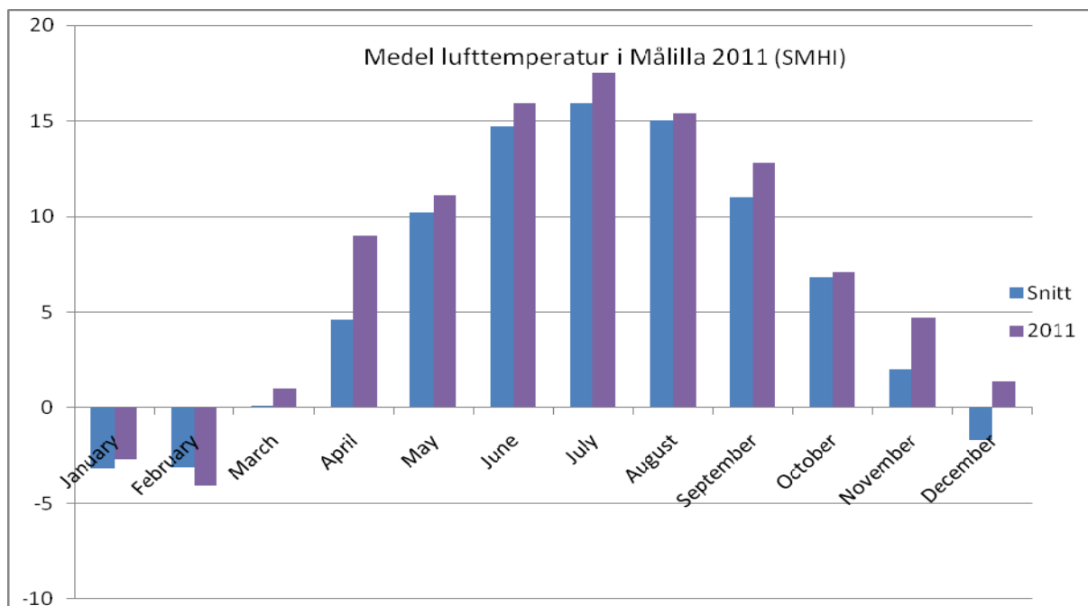
Figur 7. Medeltemperatur i Målilla 2011 enligt SMHI. (Snitt 1961 – 1990)
