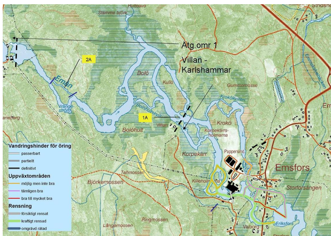
Figur 5. Översiktskarta på åtgärdsområde 1 med resultatet från biotopkarteringen 1998 samt åtgärdsträckor och åtgärdslokaler. Gränserna för projektering och åtgärdsförslag framgår med svarta, streckade linjer (Källa: www.gis.lst.se , länsstyrelsen i Jönköping 1999).
