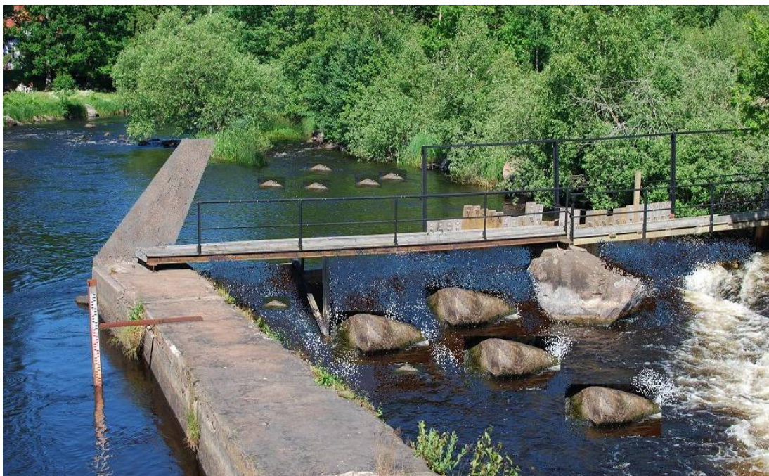
Figur 40. Retuscherad skiss på förslag på fiskväg vid åtgärdslokal 3E. Dammvallen förlängs ut till holmen och hindret rivs ut, i ovankant skapas en naturlig strömnacke och denna nivå reglerar vilket flöde som skall rinna i strömfåran.
