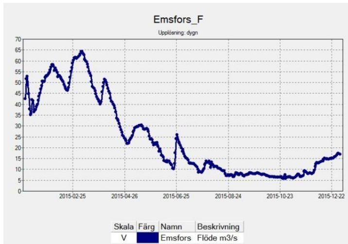
Figur 2. Emåförbundets flödemätning (m³/s) vid Emsfors.
