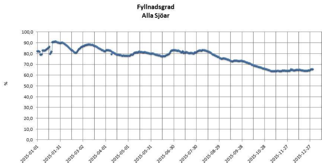
Figur 1. Fyllnadsgrad (%) samanslagna sjöar- Bellen, Hjortesjön, Flen, Hulingen, Maren, Saljen och Solgen 2015.
