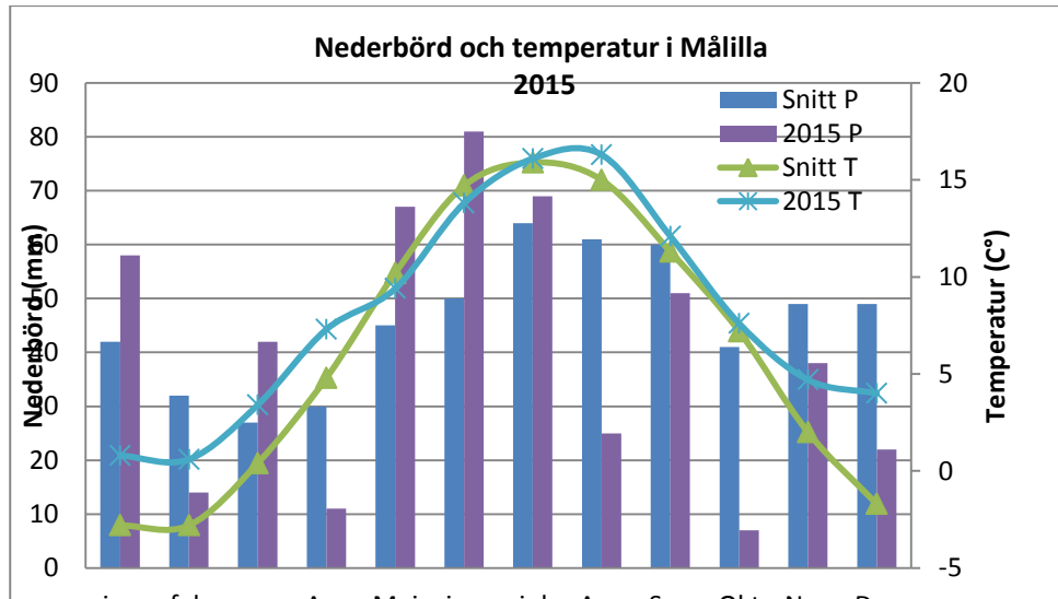
Figur 1. Nederbörd (P) och medellufttemperatur (T) i Målilla 2015 enligt SMHI (snitt 1961-1990).
