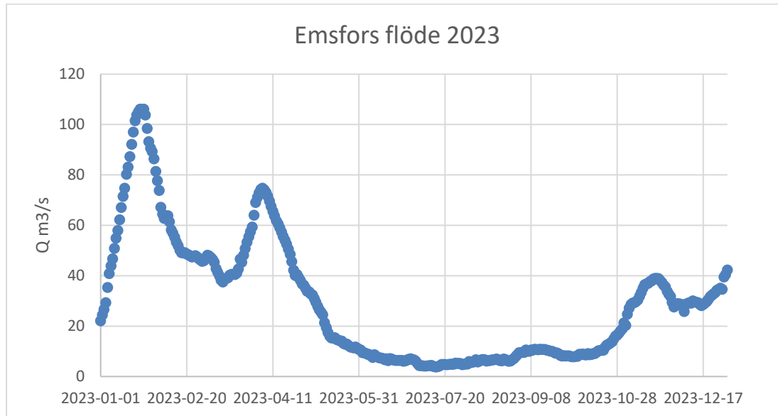
Figur 12. Flödesdata (m 3 /s) för Emsfors under 2023. Källa SCMS.
