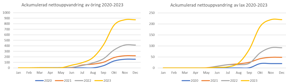
Figur 15. Diagram över uppvandrande havsöring och lax förbi Karlshammars vattenkraftverk 2020-2023.
