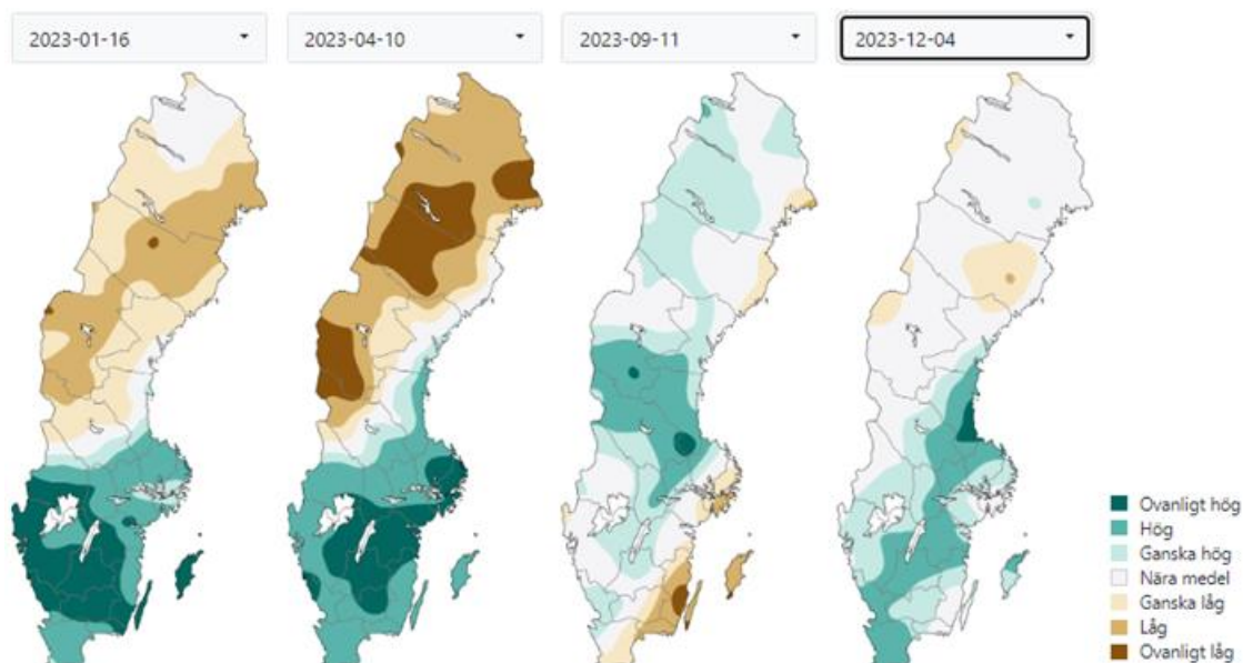
Figur 13. Grundvattennivåer i förhållande till de normala för årstiden i små grundvattenmagasin i januari, april, september och december 2023. Källa: Sveriges Geologiska Undersökning (SGU).
